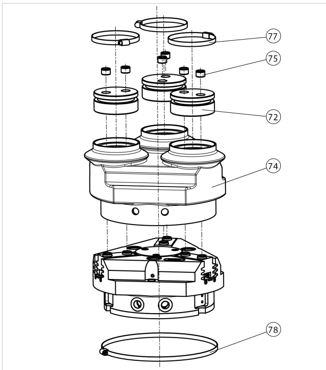
Zusammenbauzeichnung
