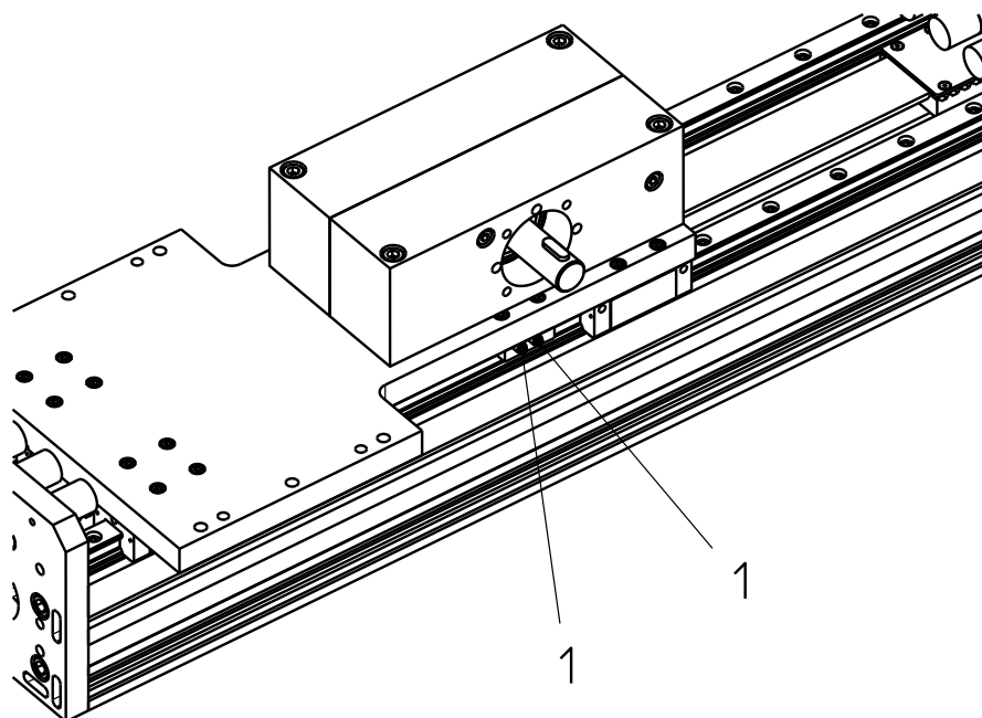
Figure 4 : Points de lubrification (1) sur le chariot
