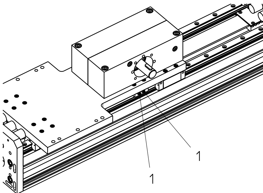
Immagine 4: Punti di lubrificazione (1) sul carrello
