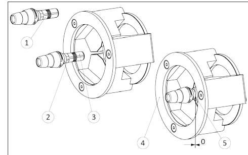
1 Druckangabe 4 SRE 2 Abflachung 5 auf Anschlag 3 Data Matrix Code
