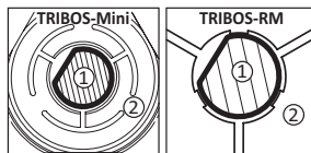
1 Schaft DIN 1835 E, DIN 6535 HE 2 Werkzeughalter
