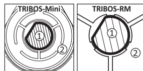
1 Shank DIN 1835 E, DIN 6535 HE 2 Toolholder
