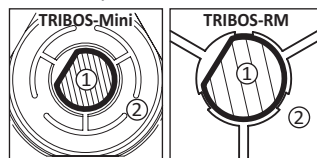
1 Shank DIN 1835 E, DIN 6535 HE 2 Toolholder
