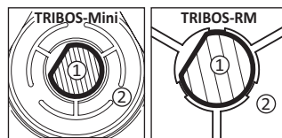
1 Schaft DIN 1835 E, DIN 6535 HE 2 Werkzeughalter
