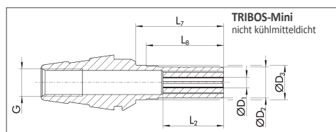
1 Schaft DIN 1835 E, DIN 6535 HE 2 Werkzeughalter
